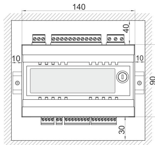
Obr. 19 Podmínky pro instalaci modulu
