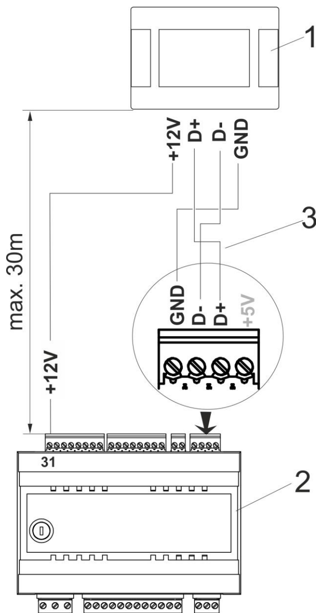
Obr. 26 Schéma elektrického zapojení (čtyřvodičového), kde: 1 – pokojový panel ecoSTER, 2 – regulátor ecoMAXX 800 R3, 3 – propojovací kabel
