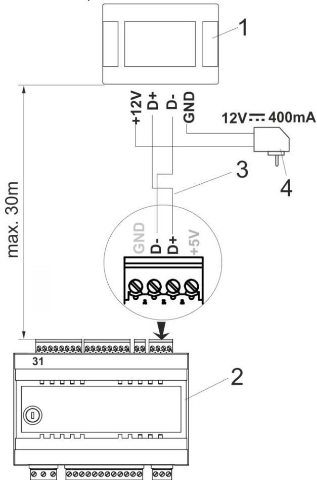
Obr. 27 Schéma elektrického zapojení (dvouvodičového), kde: 1 – pokojový panel ecoSTER, 2 – regulátor ecoMAXX 800 R3, 3 – propojovací kabel, 4 – napájení 12V.
